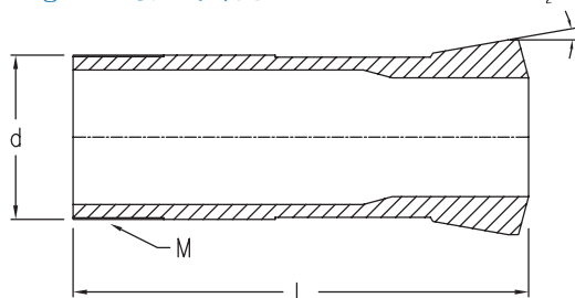
Fig. 1 後拉式筒夾
