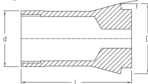
Fig. 2 前推式筒夾
